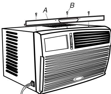
A. Top channel
