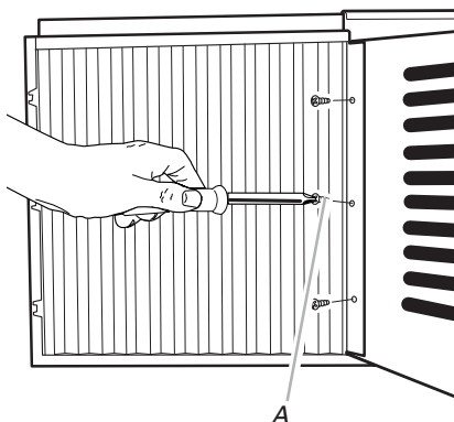
A. Tornillos de cabeza plana #8 x \frac{3}{8} "
